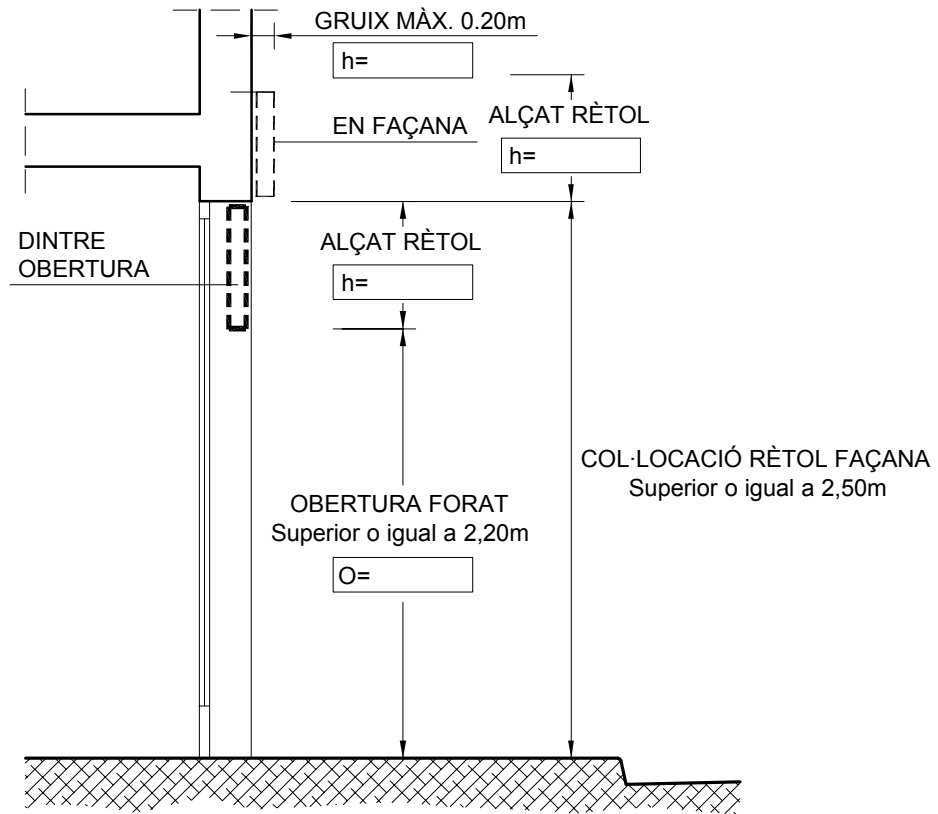
SECCIÓ
